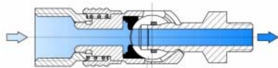
Abb. 2: Moderne Schnellkupplung
